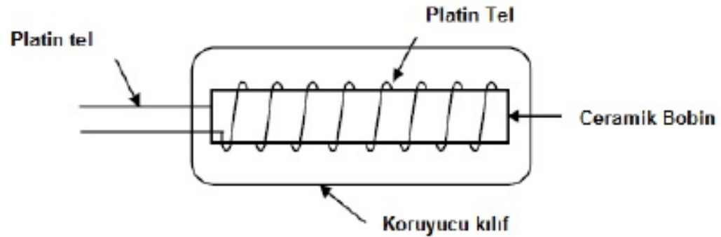
Tipik bir RTD – resistance temperature detectors
