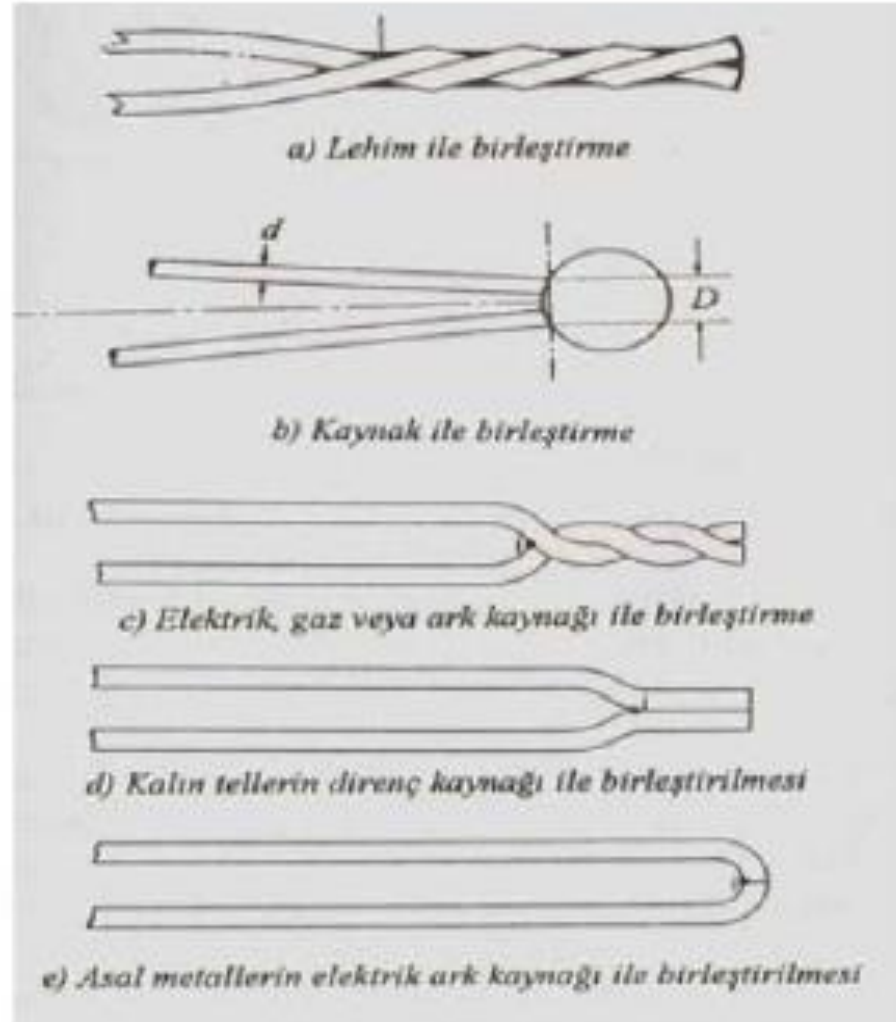
Şekil 1.5: Termokupol uçlarının birleştirilme şekillerine örnekler
