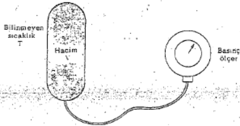
Şekil 5.18 Şematik ideal gaz termometresi.
