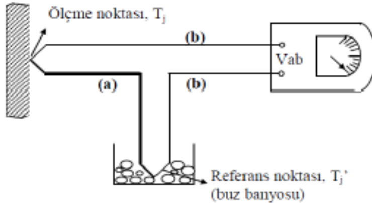
Şekil 5. Sıcaklık ölçümü için basit ısı çift devresi
